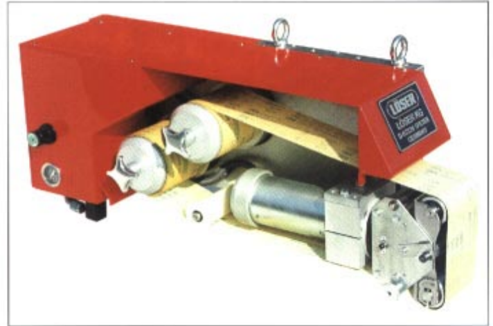
SF 102 Ausführung mit Kontakttriemen SF 102 version with contact belt
