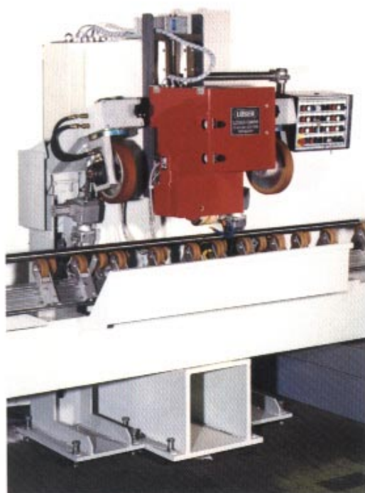
Spitzenlose Bearbeitung von Kolbenstangen Centreless finishing of cylinder rods
