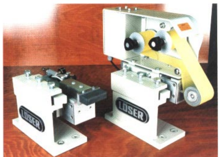
SF 105 zur Bearbeitung mit Filmen und Honsteinen SF 105 for finishing with film and hone stone
